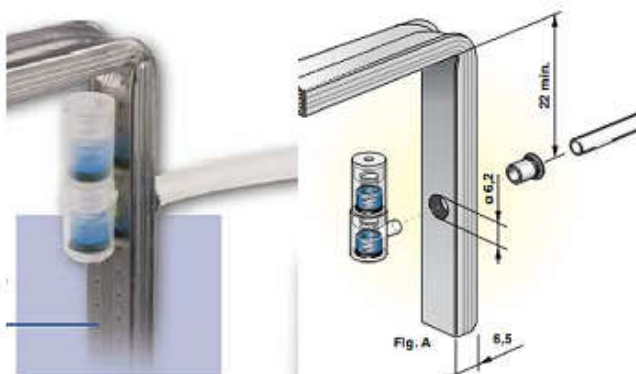
9 pav. Slėgio vožtuvo montavimas į stiklo paketą
