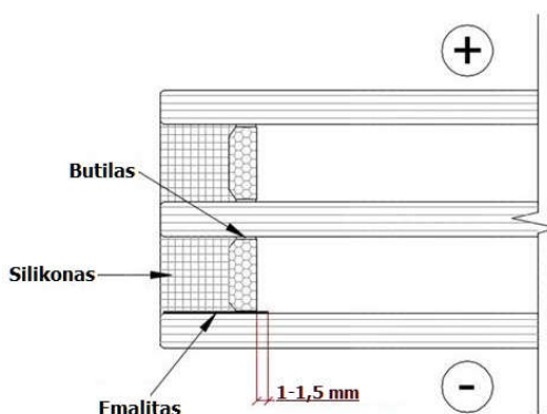
22 pav. Emaliavimo zona struktūriniam stiklinimui skirtiems stiklo paketams
