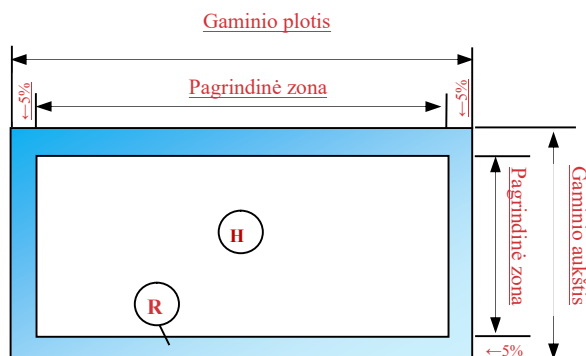
20 pav. Stiklo paviršiaus zonos tikrinimo metu
