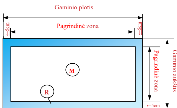
10 pav. Stiklo paketo su žaliuzėmis vertinimo zonos
