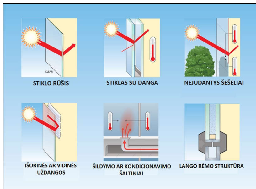
30 pav. Veiksniai įtakojančys terminio trūkio riziką
