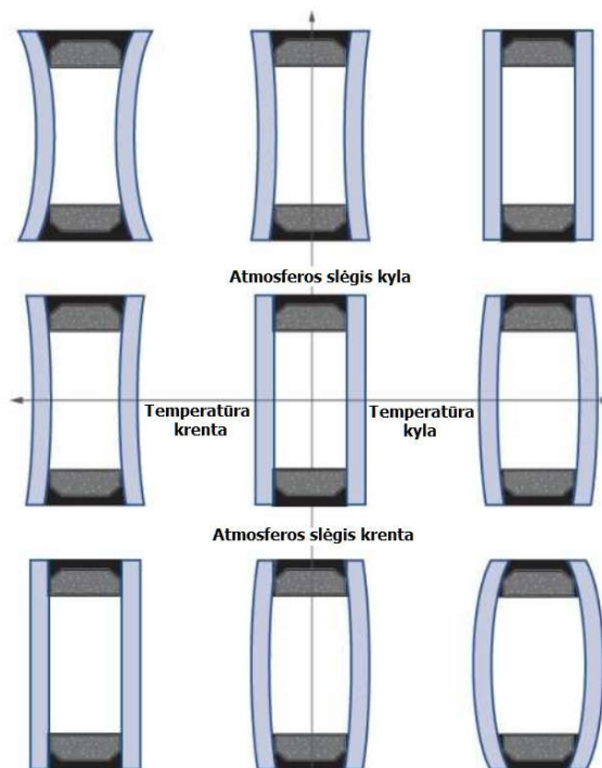
23 pav. Stiklų įsigaubimas/išsigaubimas priklausomai nuo temperatūros ir atmosferos slėgio
