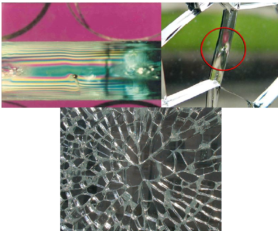
31 pav. Spontaniškos stiklo skilimo pradžia
