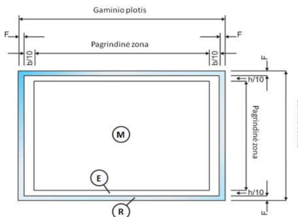
4 pav. Stiklo paketo zonos tikrinimo metu
