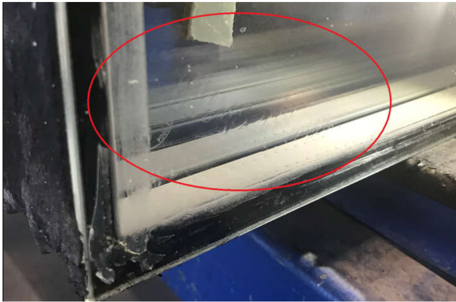
28 pav. PVB plėvelės išsilaminavimas dėl cheminio nesuderinamumo
