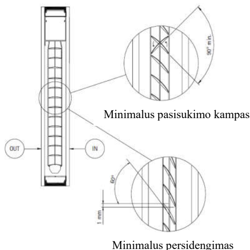
16 pav. Juostelių persidengimas
