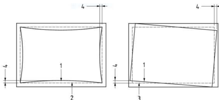
5 pav. Galimi rėmelio netolygumo variantai (1 – rėmelis, 2,3 – teorinė rėmelio priklijavimo pozicija ir forma, 4 – deviacija)
